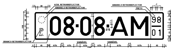
Modelo I — Automóveis (frente e retaguarda)
