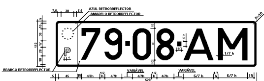
Modelo I — Automóveis (frente e retaguarda)
