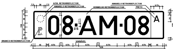
Modelo VIII — Máquinas industriais e máquinas industriais rebocáveis (frente, retaguarda ou lateral)
