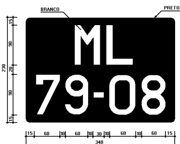
Modelo II — Automóveis (retaguarda)
