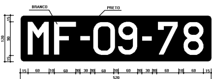
Modelo III — Automóveis (retaguarda)
