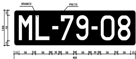
Modelo I — Automóveis (frente)
