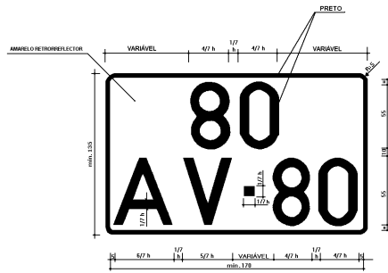
Modelo VI — Ciclomotores, motocicletas de cilindrada não superior a 50 cm 3 e quadriciclos
