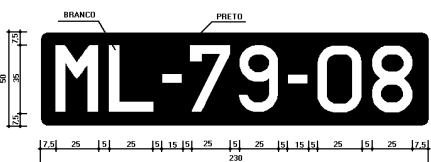
Modelo IV — Motociclos
