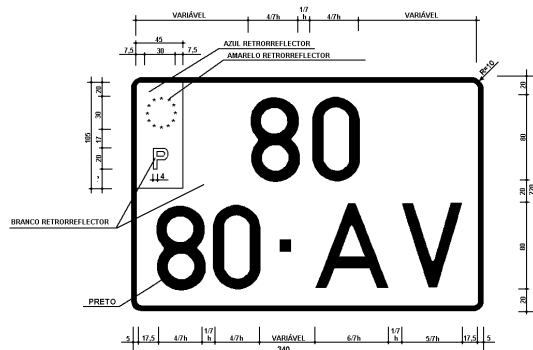
Modelo II — Automóveis (retaguarda)
